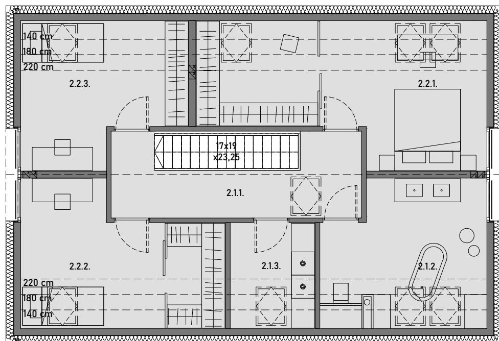
poddasze
